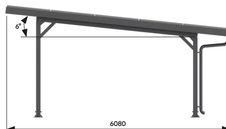
Zijaanzicht
