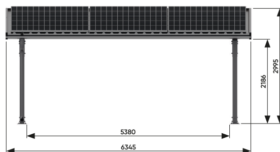
Vooraanzicht: Double
